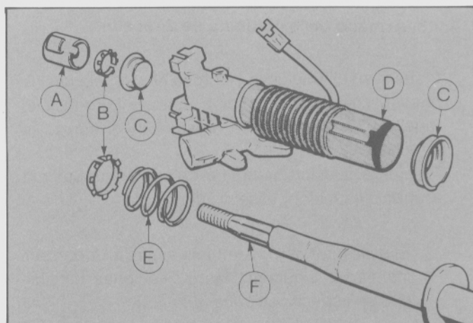
Fig. 25 - Conjunto de tubo de columna dirección.
