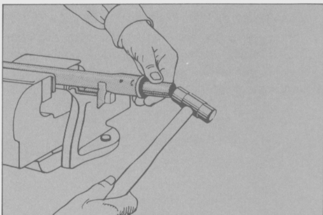
Fig. 9 - Instalación del buje guía de la cremallera.
