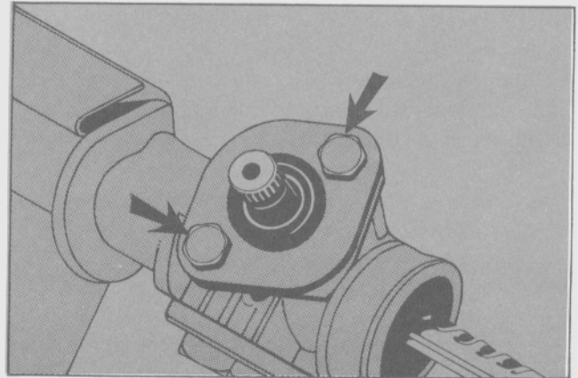
Fig. 18 - Desmontaje de la tapa del piñón.
