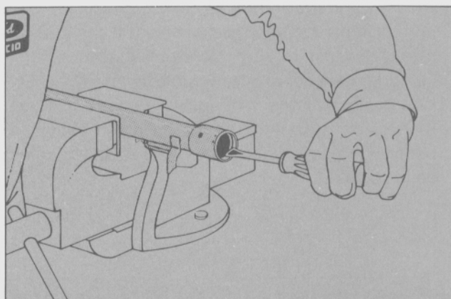
Fig. 8 - Desmontaje del buje de la cremallera.
