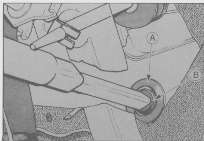
Fig. 5 - Extremo inferior de la columna A. Bujes para evitar la entrada de agua B. Bujes de eje de la dirección
