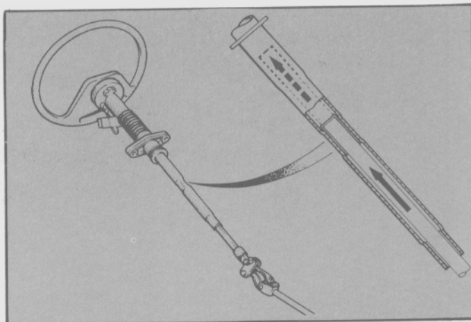
Fig. 4 - Sección plegable del eje de la dirección.
