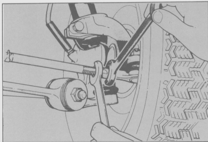
Fig. 3 - Ajuste de la convergencia
