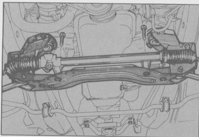
Fig. 2 - Montaje de la caja de dirección al travesaño
