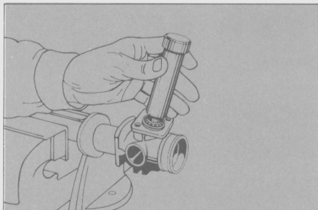
Fig. 10 - Instalación del cojinete inferior del piñón.
