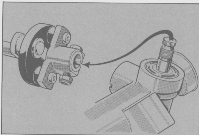
Fig. 3 - Posicionado de la junta flexible.
