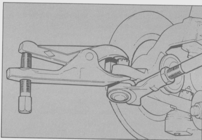
Fig. 1 - Extracción de la rótula.
