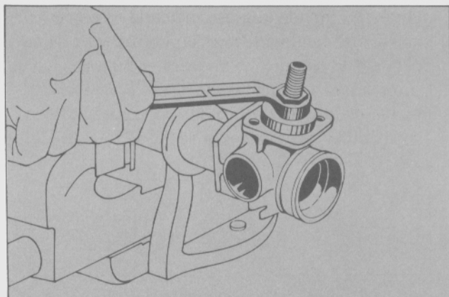
Fig. 7 - Extracción del cojinete inferior.
