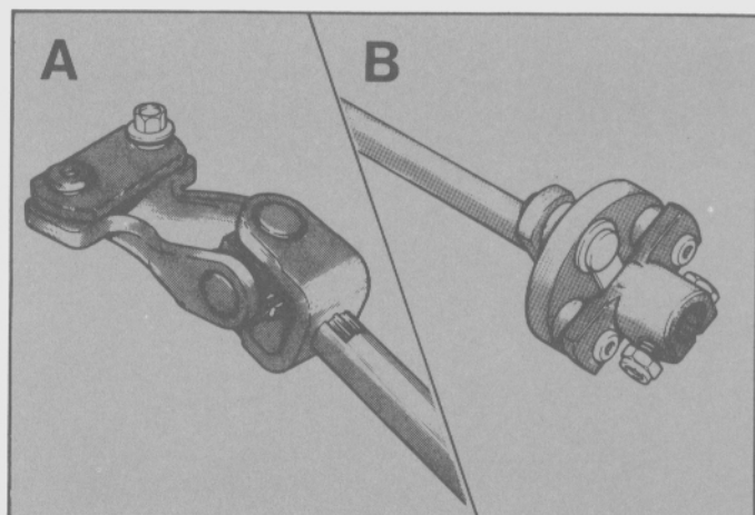
Fig. 7 - A. Junta universal B. Acoplamiento elástico
