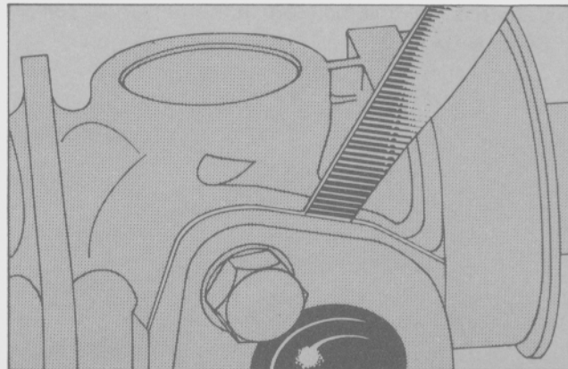
Fig. 19 - Control del huelgo de la tapa del piñón sin junta.
